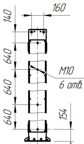
Места для крепления к турникету полноростовых ограждений «Ростов-Дон» (вид на стойки 1 и 2 справа и слева) (вид на стойки 1 и 2 справа и слева)
