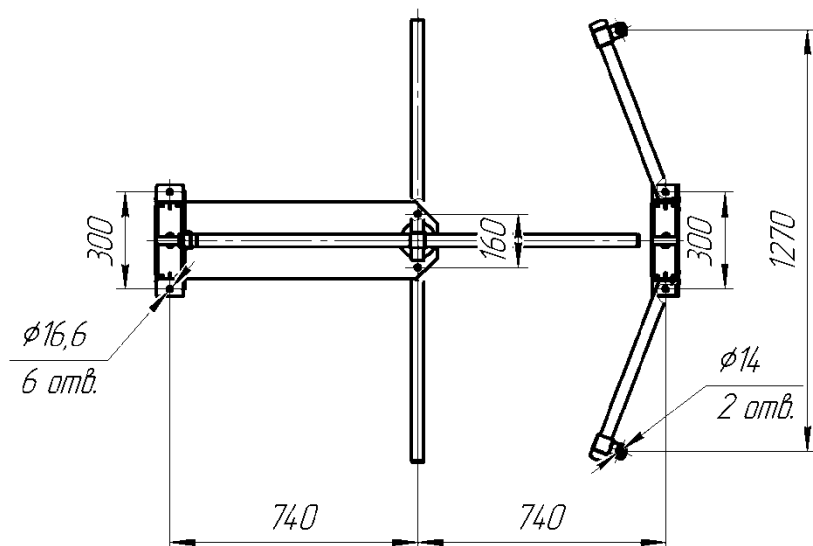
Установочные размеры турникета «Ростов-Дон ПР1Л/4М2»
