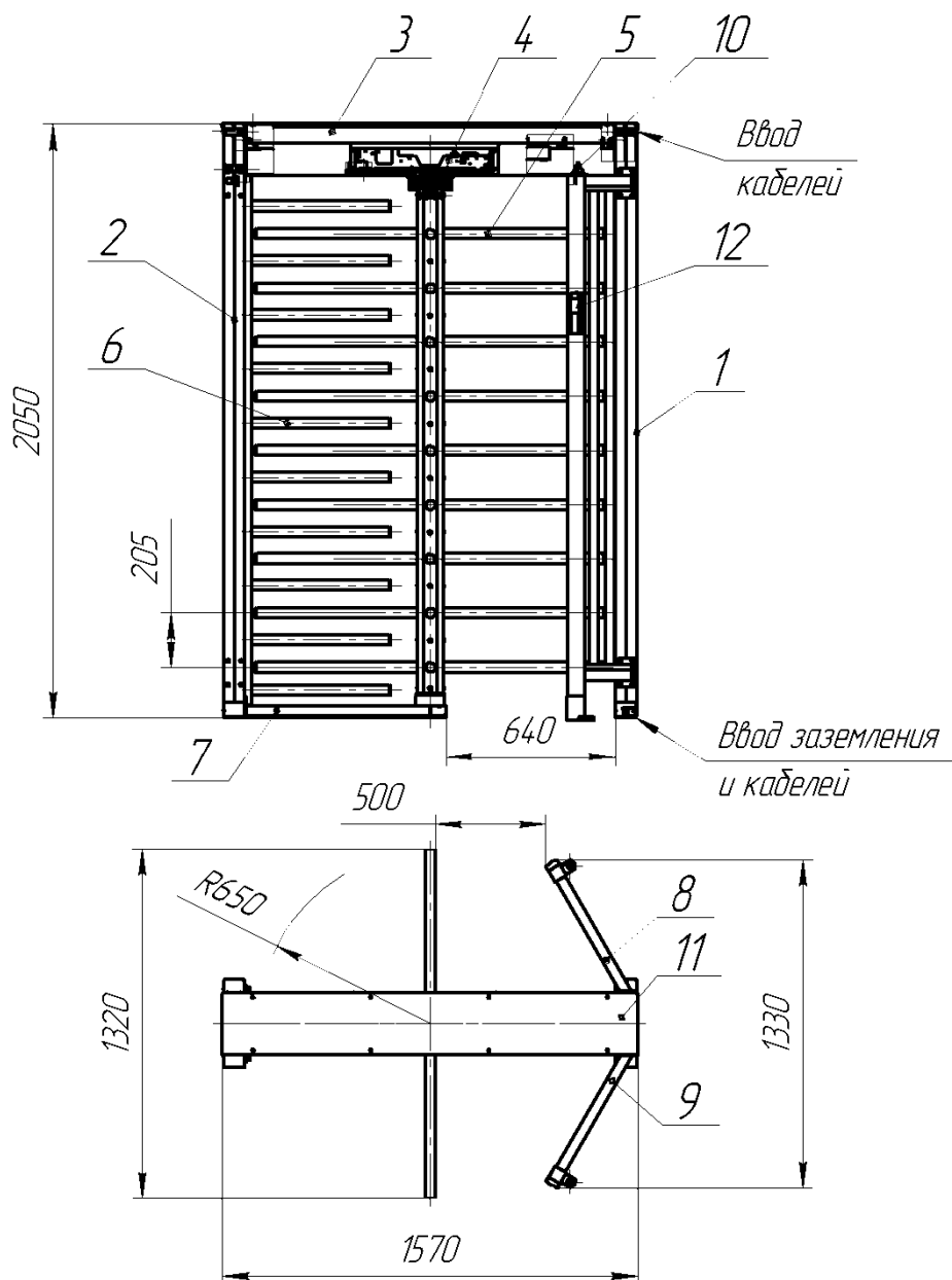
Габаритные размеры турникета «Ростов-Дон ПР1Л/4М2»
